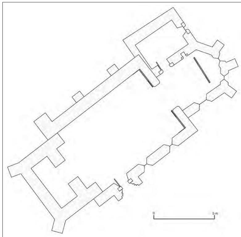
10. kép: A Solt, tételhegyi templom alaprajza, 14–16. sz.
