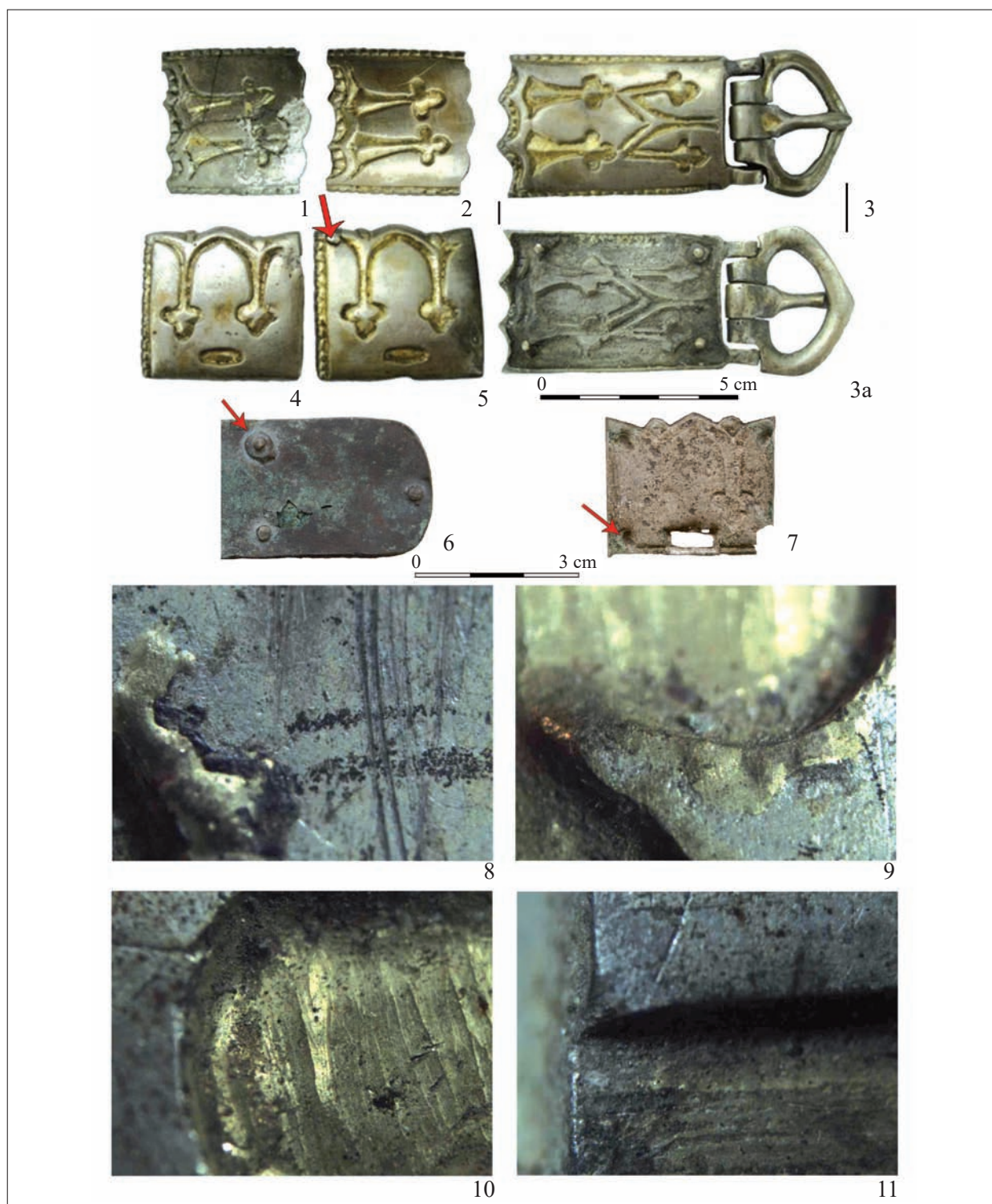
15. kép. Az övveretek vizsgálata (1–5: Karancslapujtó 1. sír; 6–11: Krjukovo-Kuzsnovo 505. sír). 5: A sérült felszerelőcsap átfűrással való javítása; 6–7: A felerősítés elemei (ellentettlemezt, illetve a felforrasztás gömb alakú nyoma); 8–9: Az aranyozás mintán túlfutó részletei; 10–11: A tüziaranyozás során végzett felület megmunkálási nyomok (megmunkálás a tüziaranyozás felvitele előtt, illetve az öntés utáni eldolgozás nyoma a peremen)
