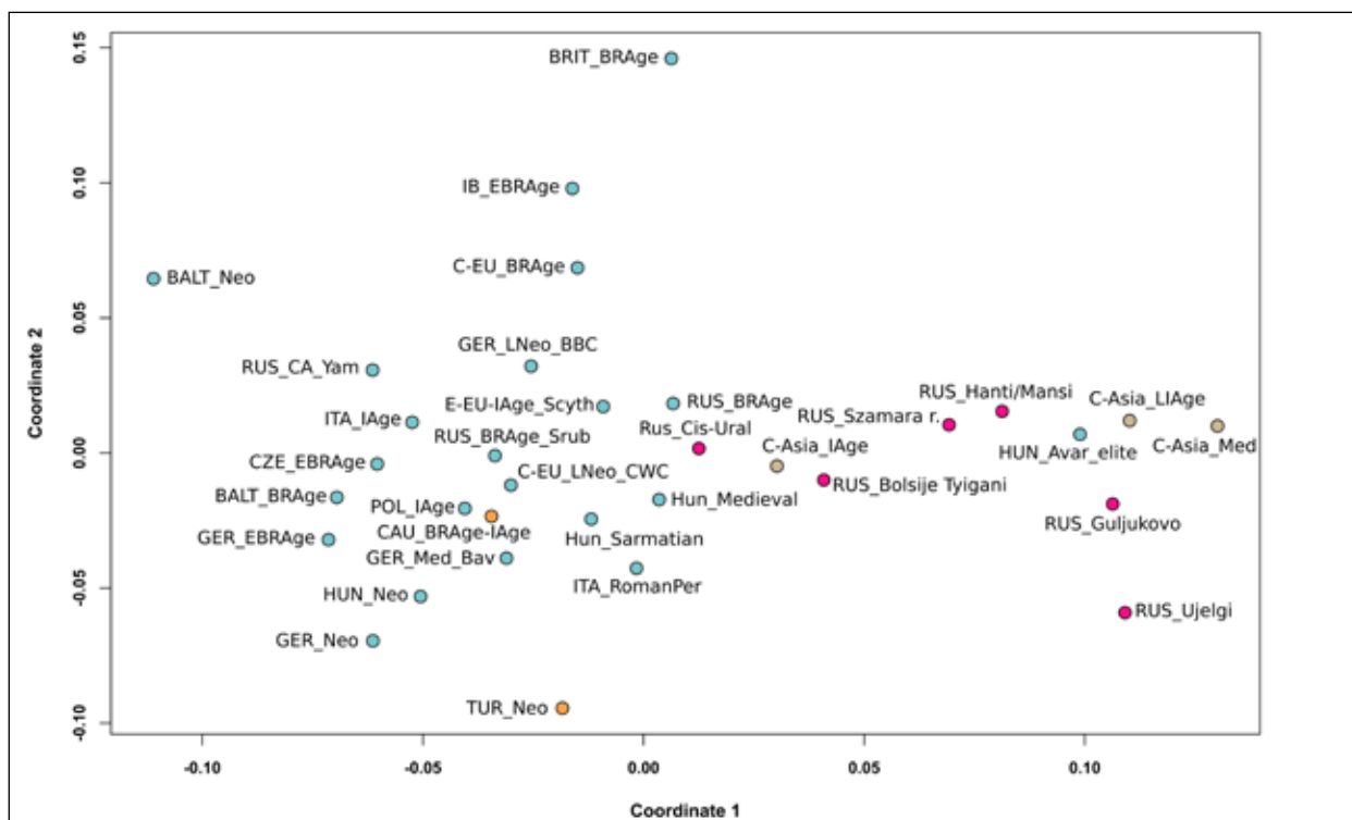
3. ábra. Archaikus populációk MDS (multidimensional scaling) plotja, amely teljes mitogenom szekvenciákból számított genetikai távolságokon alapul. Kékkel az európai, sárgával a közel-keleti barnával az ázsiai, pinkkel az általunk vizsgált populációkat jelöltük. A Cis-Ural (Urál nyugati fele) és Ujelgi (Urál keleti oldala) névvel jelölt (korai magyarokkal régészeti leletek alapján kapcsolatba hozható) populációkról ld. jelen kötetben Gerber és mtsai. cikkét. (az elemzésekhez felhasznált archaikus populációkról bővebb információ: Csáky V. et al. 2019a)
