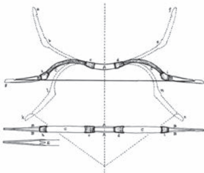
AZ ÍJ SZERKEZETE ÉS MŰKÖDÉSE Cs. SEBESTYÉN KÁROLY REKONSTRUKCIÓS RAJZÁN (1932).
