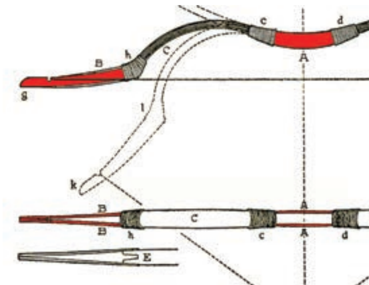
A MARKOLAT- ÉS A SZARVLEMEZEK ELHELYEZKEDÉSE AZ ÍJON.
