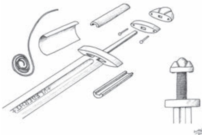
KARDMARKOLAT SZERKEZETI ÁBRÁJA.
