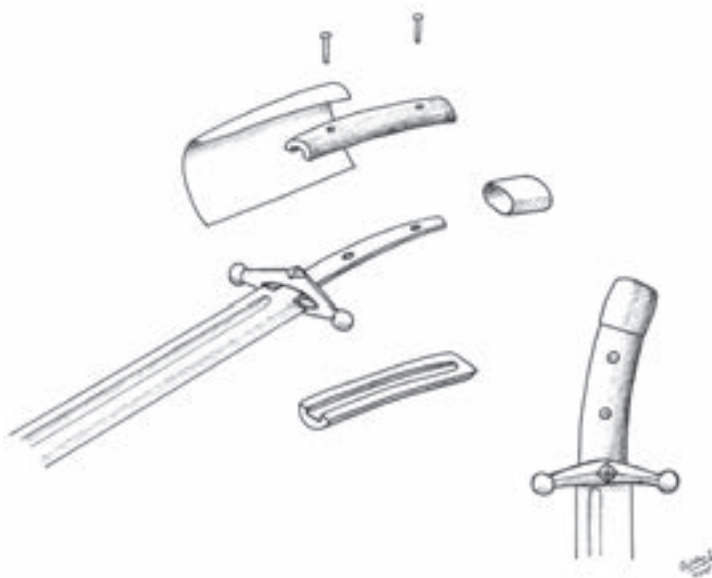
SZABLYAMARKOLAT SZERKEZETI ÁBRÁJA.
