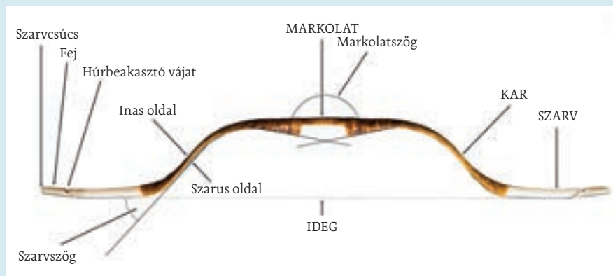
AZ ÖSSZETETT REFLEXÍJ FŐ RÉSZEI. FOTÓ: BENCSIK PÉTER
