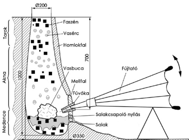
A PRÓBAKOHÓSÍTÁSOKHOZ HASZNÁLT FAJSZI TÍPUSÚ BUCAKEMENCE GEOMETRIAI MÉRTEI, FELÉPÍTÉSE ÉS A KÍSÉRLETEK ELRENDEZÉSI VÁZLATA
