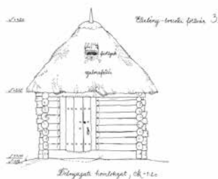
BORONAHÁZ RAJZI REKONSTRUKCIÓJA. SABJÁN TIBOR MUNKÁJA
